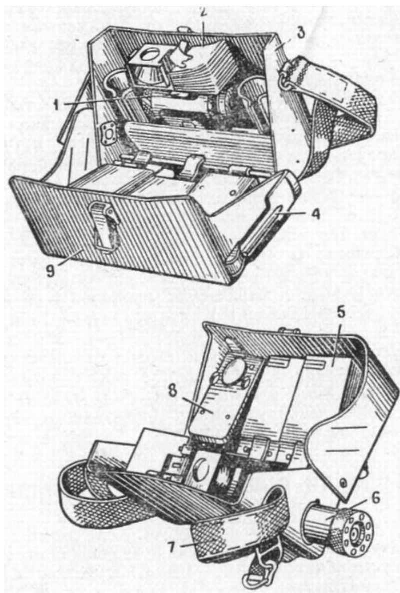
Рис. 9.20. Прибор химической разведки: 1 - насадка к насосу; 2 - противодымные фильтры; 3 - корпус; 4 - лопатка; 5 - кассеты с индикаторными рубками; 6 - ручной насос; 7 - плечевой ремень; 8 - электрический фонарь; 9 - крышка
